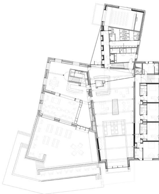
Plan du rez supérieur
